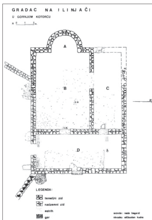
Nacrt plana kasnoantičke crkve iz Graca u Gornjem Kotorcu (prema: Fekeža, 1990. Plan II)
